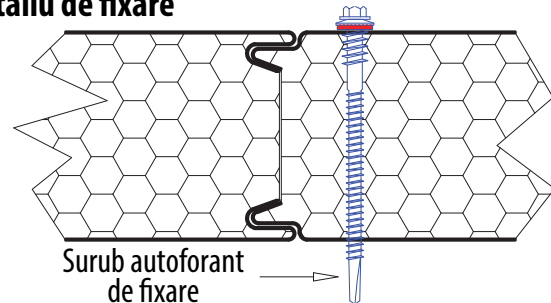
profil micro-nervurat
